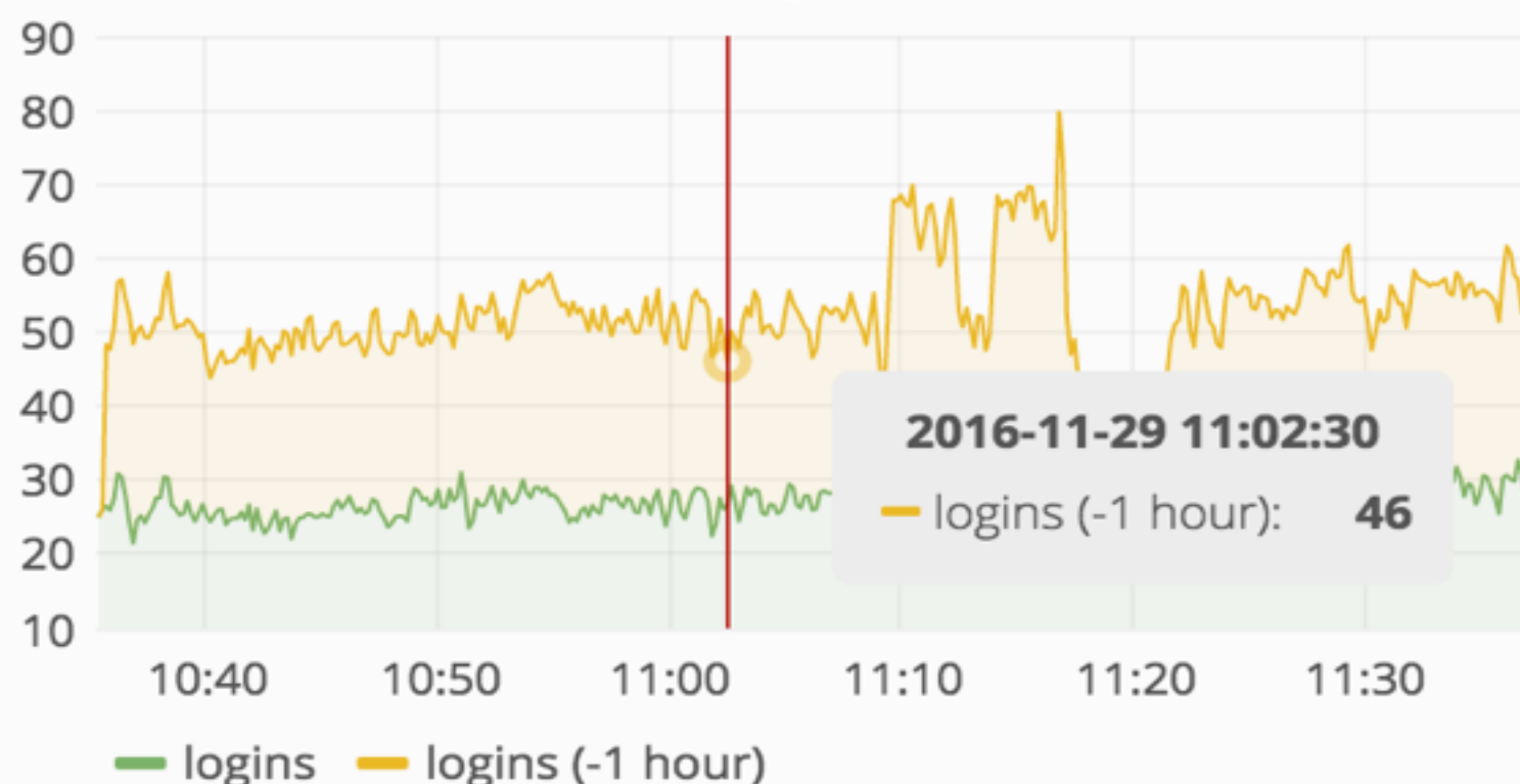
logins
